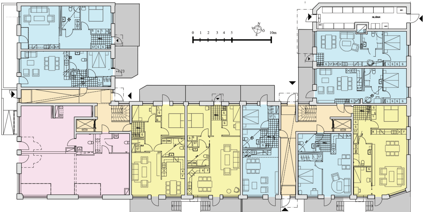
entréplan
